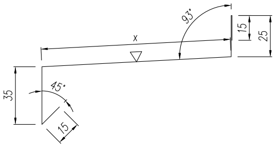
Alsó vízszintes ablak szegély
