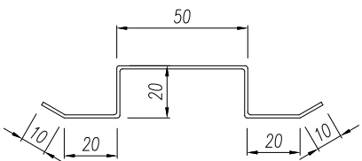
Közbenső profil 20/50
