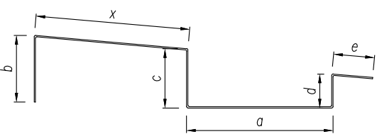
Attika szegély támasza
