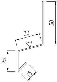
Indító profil
