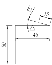
Homlokzati toldó elem más elemmel való összekapcsoláshoz
