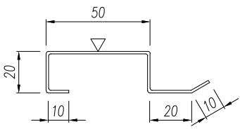
Záróprofil 20/50
