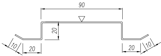
Alapprofil 20/90
