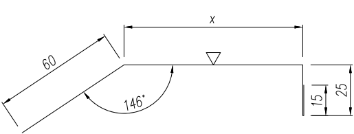
Felső vízszintes ablak szegély
