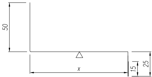
Függőleges ablak szegély
