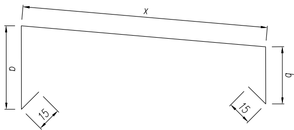
Attika szegély
