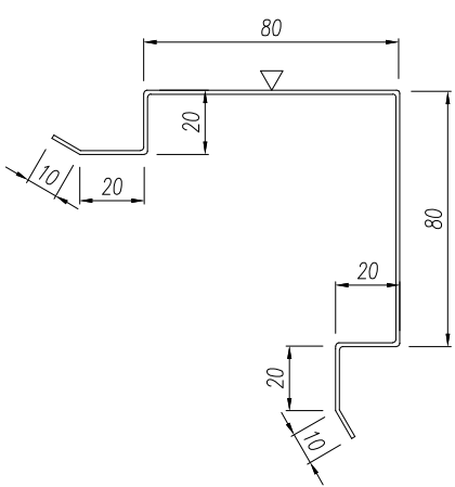
Sarokprofil 20/160
