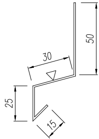
Indító profil
