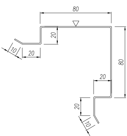
Sarokprofil 20/160
