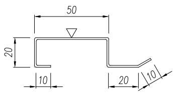
Záróprofil 20/50
