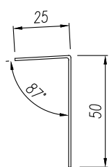
Alsó vízszintes ablak szegély támasza
