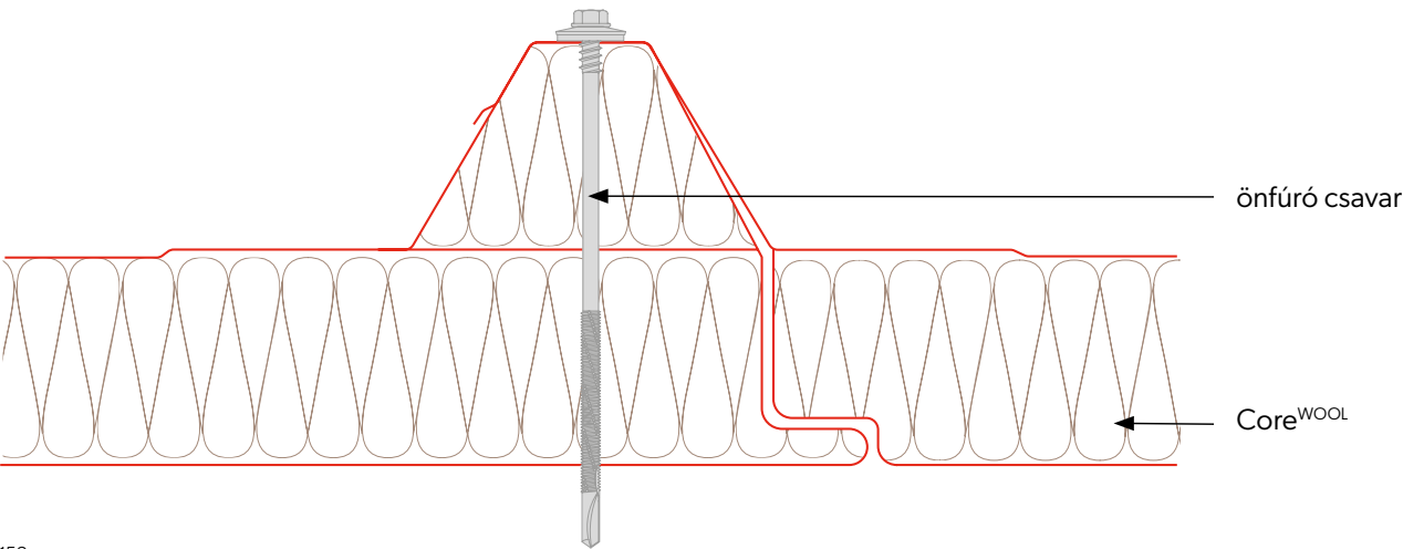
Szendvicspanelek összeillesztése
