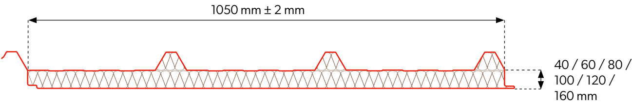
Födém keresztmetszet
