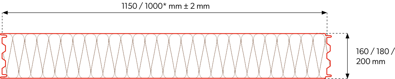
Födém keresztmetszet
