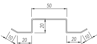
Közbenső profil 20/50
