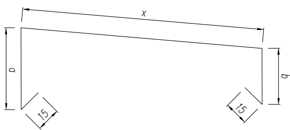
Attika szegély
