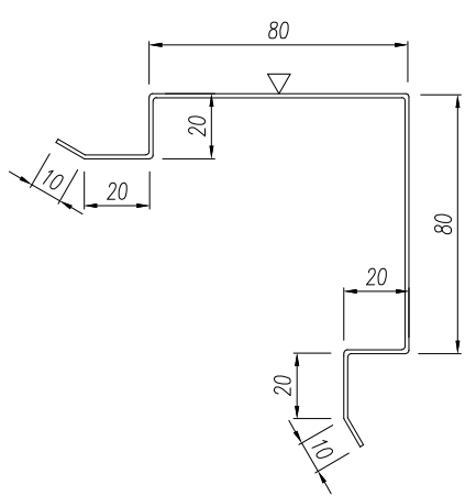
P04 Sarokprofil 20/160
