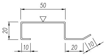
P02 Záróprofil 20/50
