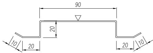
P03 Alapprofil 20/90
