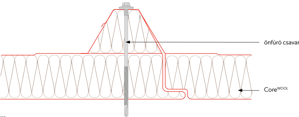
Szendvicspanelek összeillesztése
