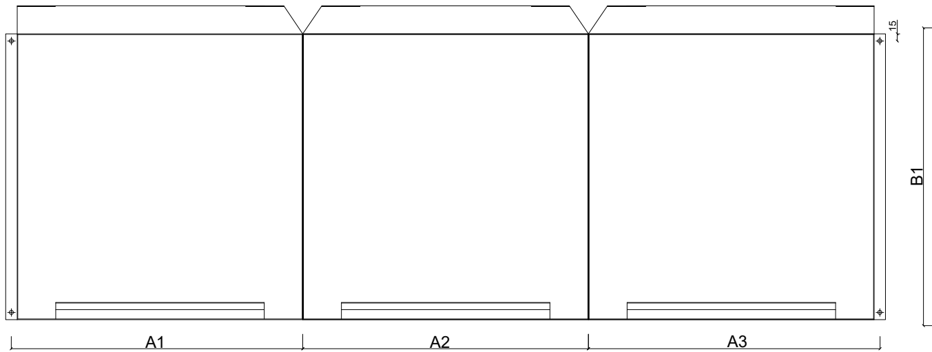
Rohový systém U na montáž vo zvislom systéme. A1max + A2max + A3max = 3000 mm, A1min = 300 mm, A2min = 300 mm B1min = 300 mm, B1max = 800 mm, B1min = 300 mm, B1max = 800 mm
