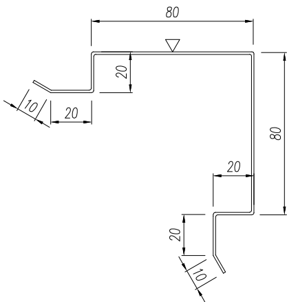
P04 Profil rohový 20/160
