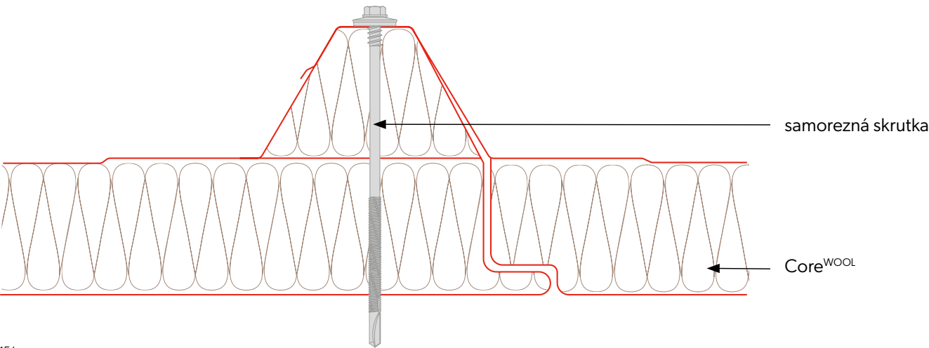
Spájanie panelov
