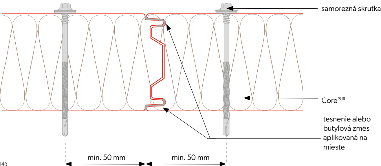
Spájanie panelov
