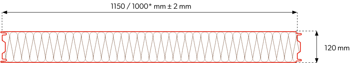
Spájanie panelov
