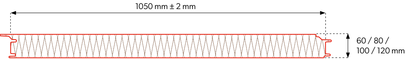
Prierez panela
