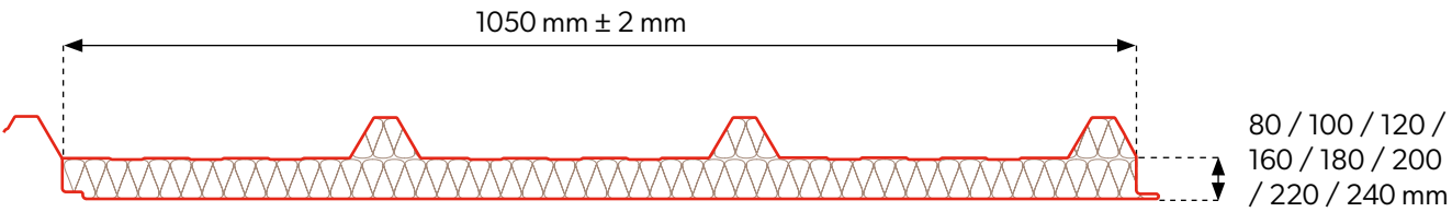
Prierez panela
