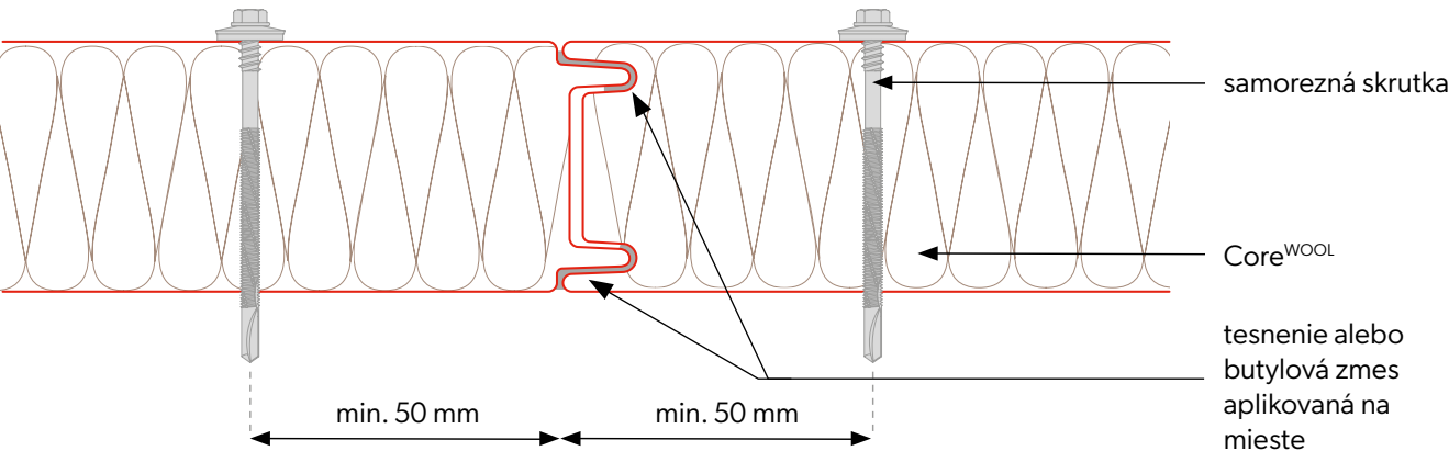
Spájanie panelov
