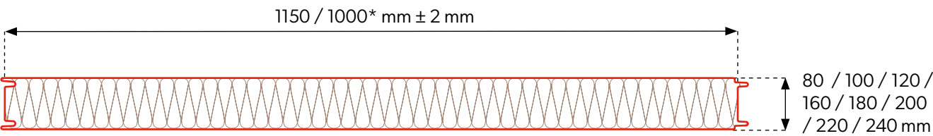
Prierez panela
