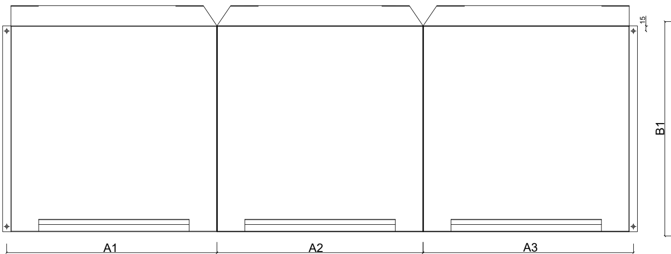
Panou de colț în formă de U pentru instalare verticală. A1_{max} + A2_{max} + A3_{max} = 3000\text{ mm} , A1_{min} = 300\text{ mm} , A2_{min} = 300\text{ mm} B1_{min} = 300\text{ mm} , B1_{max} = 800\text{ mm} , B1_{min} = 300\text{ mm} , B1_{max} = 800\text{ mm}
