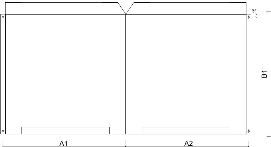
Panou de colț în formă de L pentru instalare verticală. A1_{max} + A2_{max} = 3000\text{ mm} , A1_{min} = 300\text{ mm} , A2_{min} = 300\text{ mm} B1_{min} = 300\text{ mm} , B1_{max} = 800\text{ mm}
