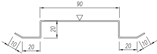
P03 profil de bază 20/90
