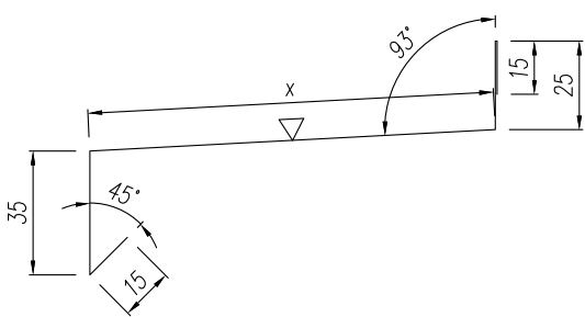
O05 Orizontal fereastră de jos intermitent
