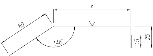
O04 Element orizontal pentru fereastră, nivel inferior
