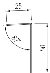
O06 Suport orizontal pentru jaluzelele de jos ale ferestrei
