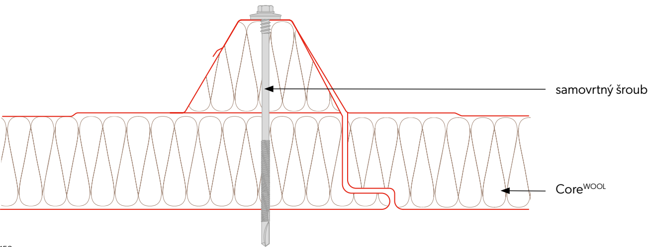
Upevnění panelů
