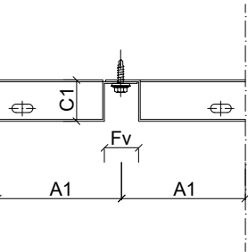
Svislé spojení
