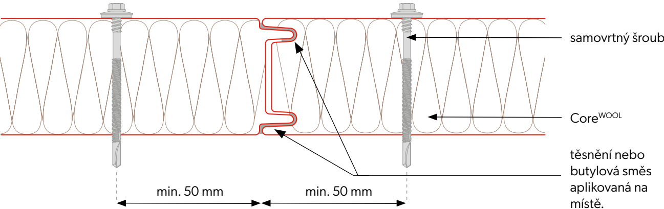
Upevnění panelů
