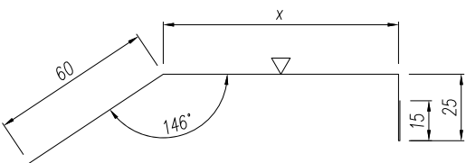
O04 Vodorovné horní zpracování okna
