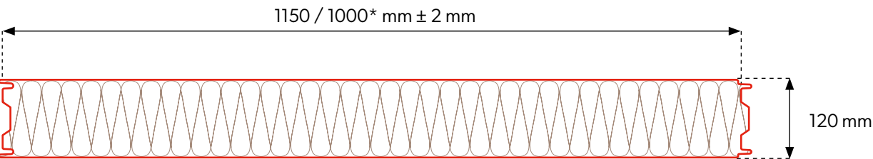
Szendvicspanelek összeillesztése
