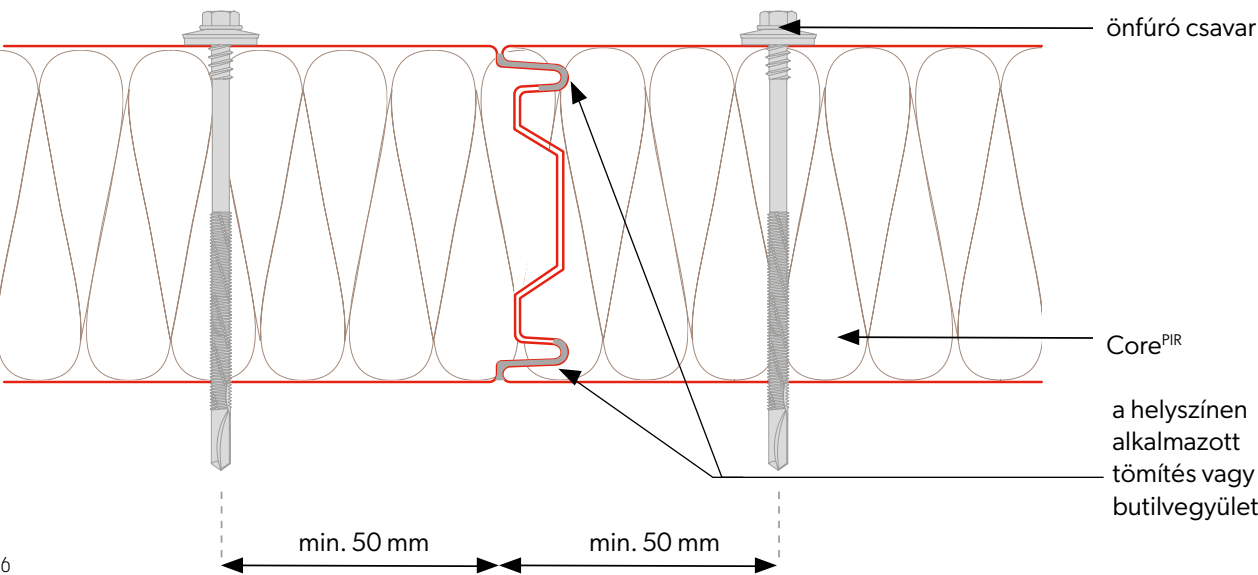
Szendvicspanelek összeillesztése
