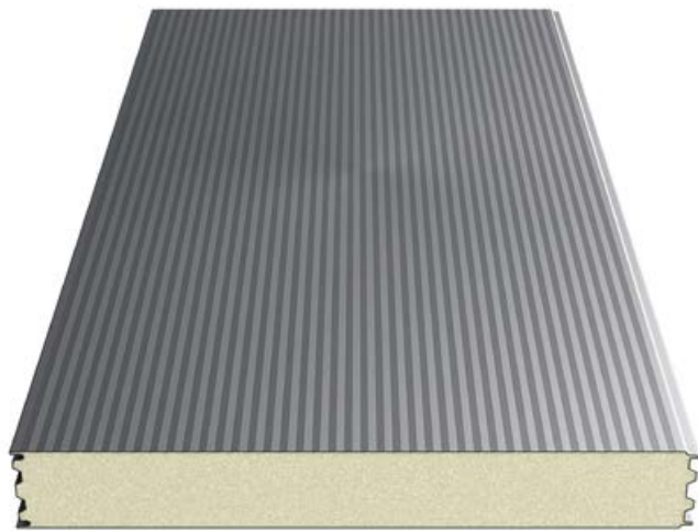
Födém keresztmetszet
