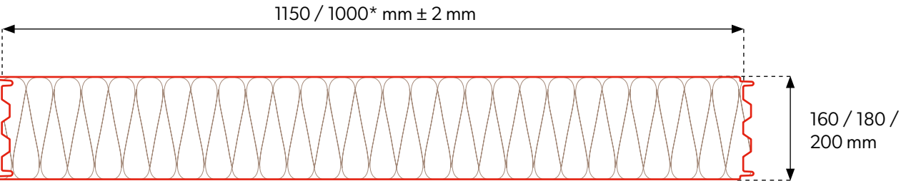
Szendvicspanelek összeillesztése
