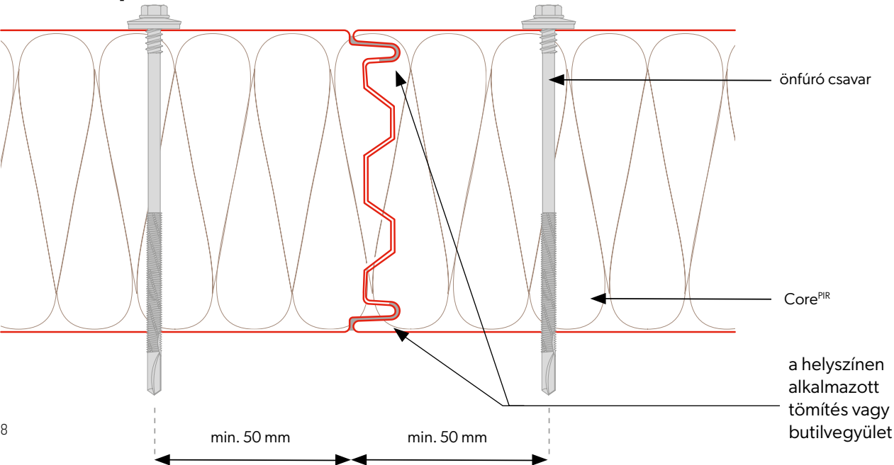
Szendvicspanelek összeillesztése
