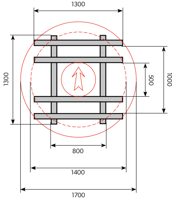
Paleți pentru fâșii cu un diametru de la 1400 mm la 1700 mm.
