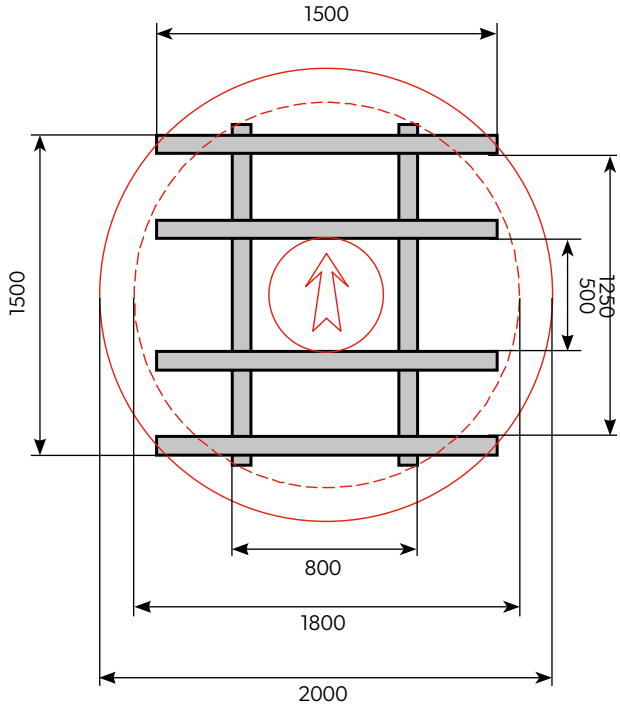
Paleți pentru fâșii cu un diametru de la 1700 mm la 2000 mm.
