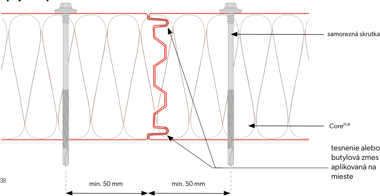
Spájanie panelov
