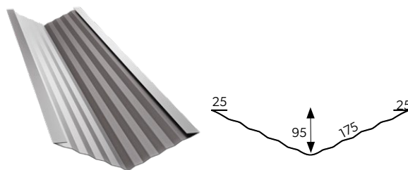
RYNNA KOSZOWA
