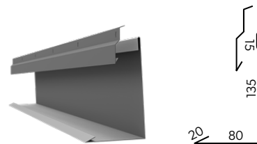
OBRÓBKA PRZYŚCIENNA Z LISTWĄ DYLATACYJNĄ
