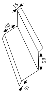
STOGO SIENOS KAMPAS I
