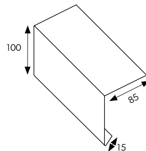
LAŠTAKIS
