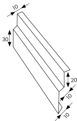
DILATACIJOS JUOSTA
