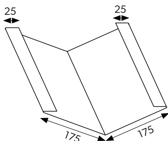
SĄLAJA
