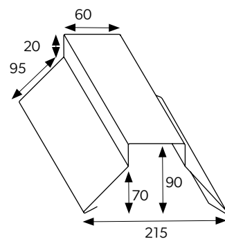
TRAPECINIS KRAIGAS
