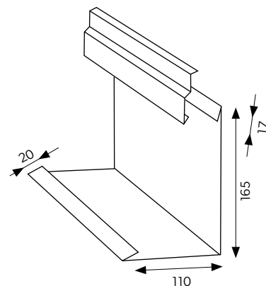
STOGO SIENOS LANKSTINYS SU DILATACIJOS JUOSTA
