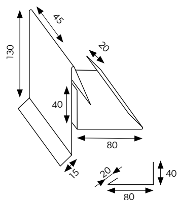
VĖJALENTĖ II
