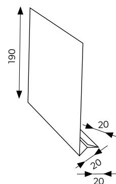
UNIVERSALUS LAŠTAKIS/ VĖJALENTĖS PRAILGINIMAS
