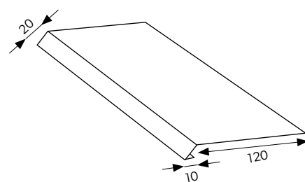
ŠLAITO JUOSTA
