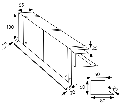
VĖJALENTĖ III
