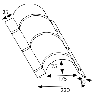
GAŚIOR BARYŁKOWY
